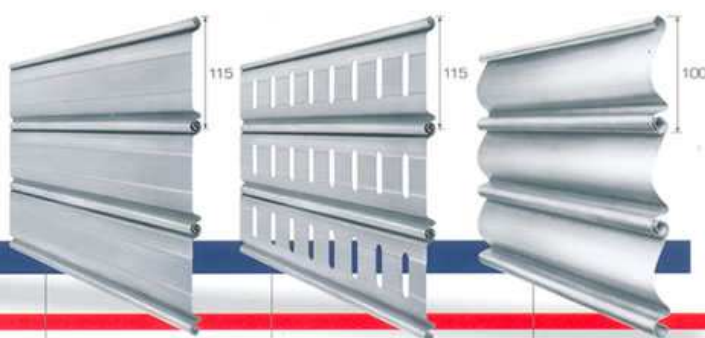
ELEMENTI CHIUSI ELEMENTI CON ASOLE DI AREAZIONE ELEMENTI PER SERRANDE DI GRANDI DIMENSIONI
